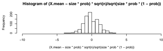
図 5: 中心極限定理の例 (二項分布の場合) ヒストグラムはそれぞれ、上段 : 元のデータ、中段 : (平均-真値)、下段 : (平均-真値) \sqrt{n}/\sigma
